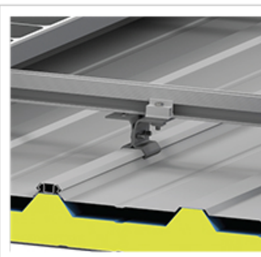
[ 모듈 부하 하중 분산 ] 태양광 구조연결부
