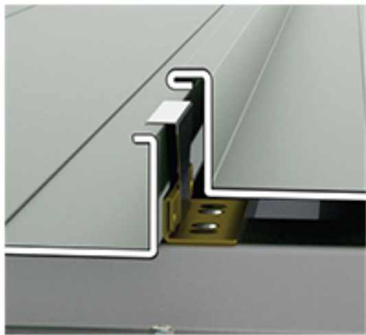
[ 누수보호 거열접기 ] 아트그린 패널
