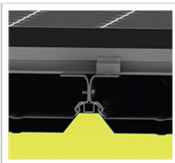
[ 거치부재 결합 ] 태양광 패널 부착
