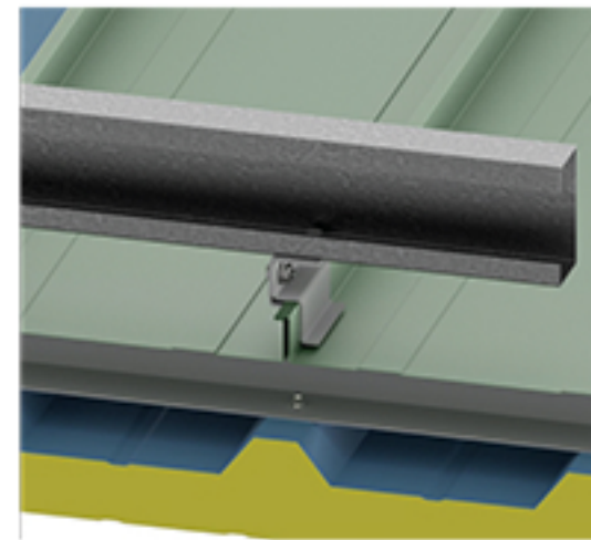
[ 모듈 부하 하중 분산 ] 태양광 구조연결부
