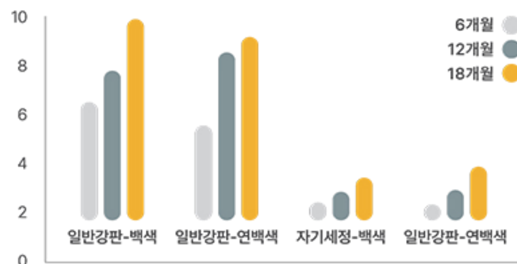
[ 자기세정 PCM과 일반 PCM의 일반폭로 시험결과 ]
