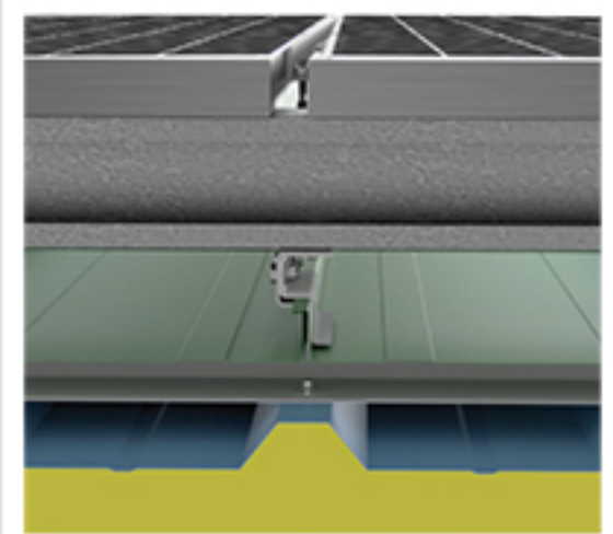
[ 거치부재 결합 ] 태양광 패널 부착
