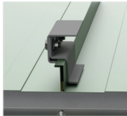
[ 지붕 변형 최소화 ] 무타공 클램프
